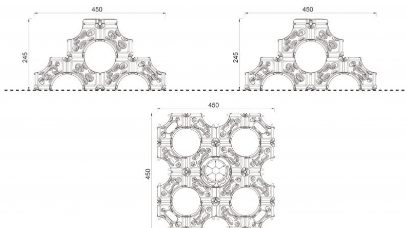
Zał. 1. Wymiary urządzenia
