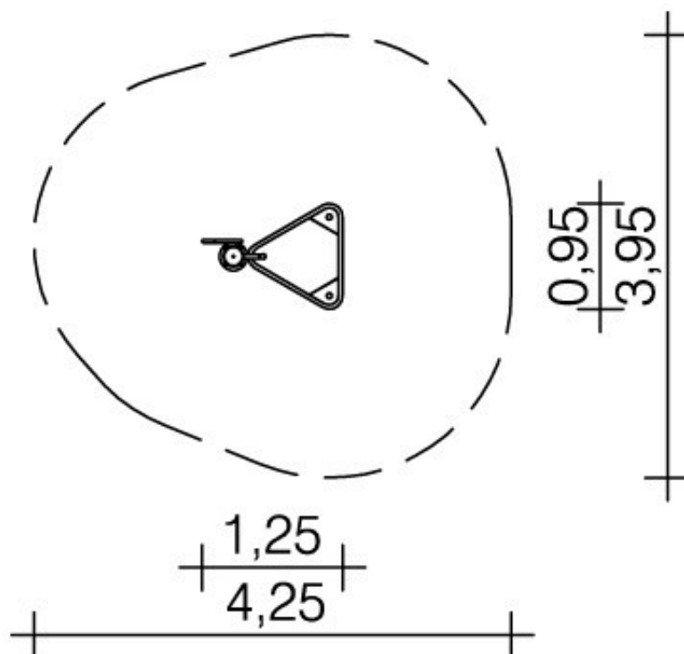
Rys. 1. Wymiary urządzenia i strefy bezpieczeństwa
