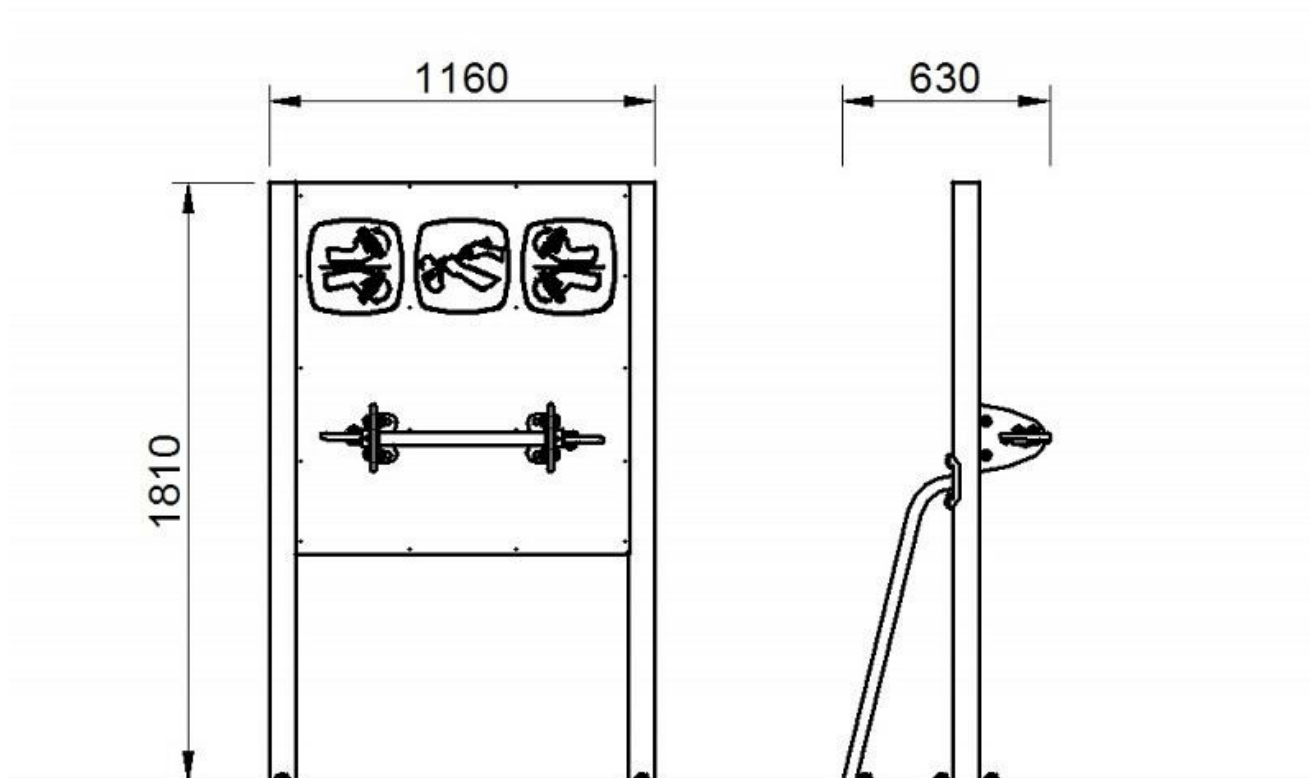
Zał. 1. Wymiary urządzenia
